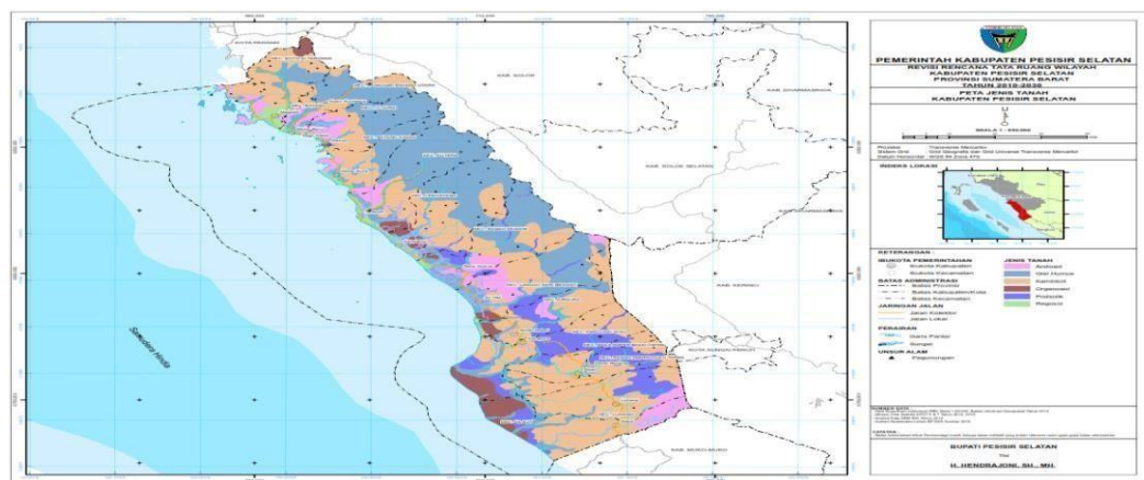
Gambar 2.6 Peta Jenis Tanah Kabupaten Pesisir Selatan
