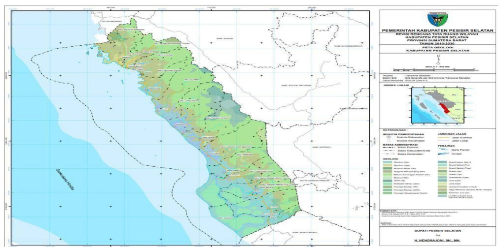
Gambar 2.5 Peta Geologi Kabupaten Pesisir Selatan
