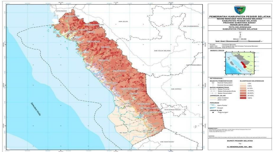
Gambar 2.3 Peta Kelerengan Kabupaten Pesisir Selatan
